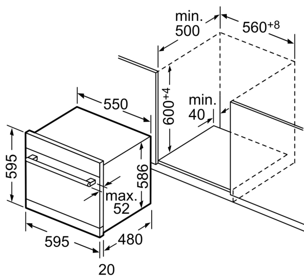
Méretetek mm-ben
